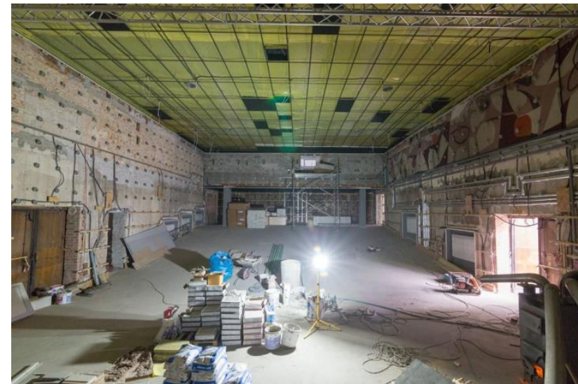
Sala widowni kinoteatru - konstrukcja pod ekofony - płyty wygłuszające
