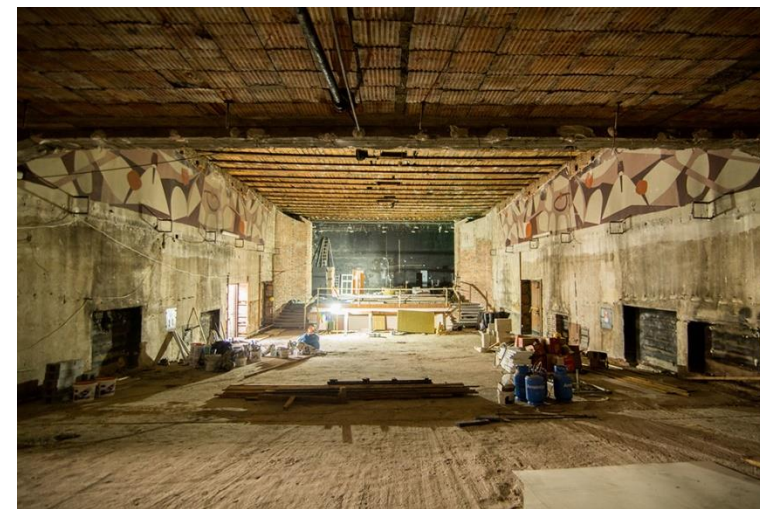
Budynek sali kinowo-widowiskowej. Roboty rozbiórkowe, demontaż sufitu podwieszanego.
